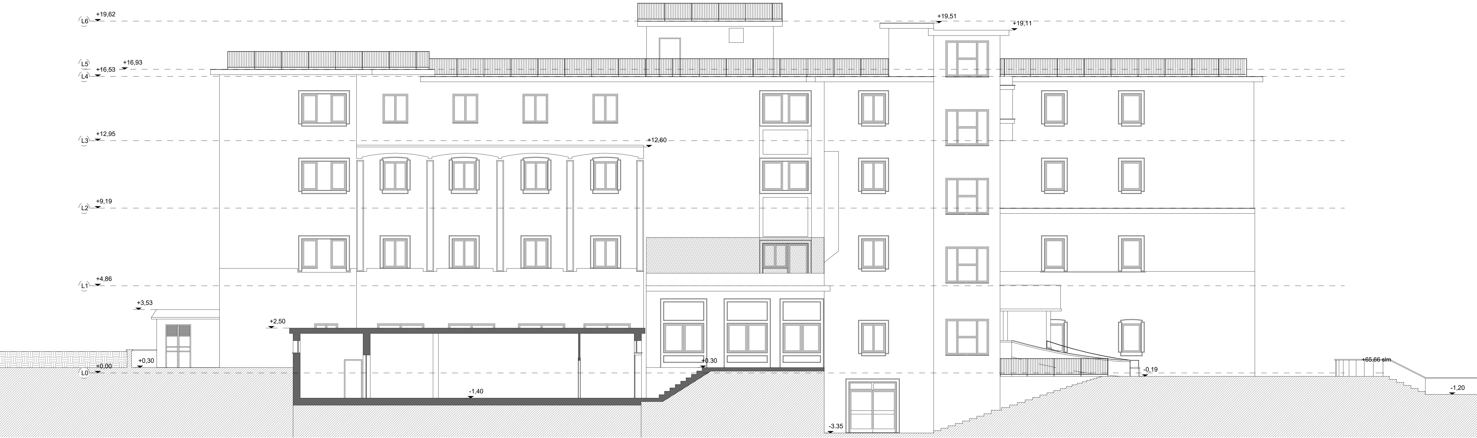
2-2 Stato di fatto - Prospetto Nord-Ovest
